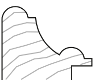
2320 (23x20 mm. - rebajo 6x4 mm.)
