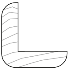
G28 (28x28 mm. - rebajo 20x20 mm.)
