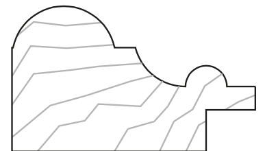
4728 (47x28 mm. - rebajo 8x8 mm.)
